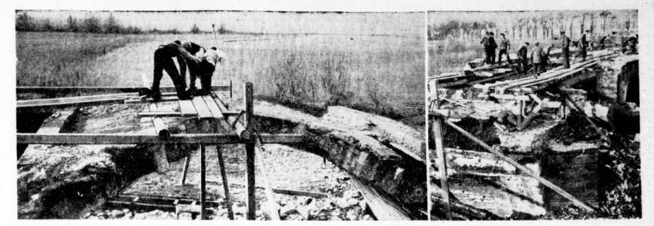
Ein Bogen unmittelbar vor der „Sprengung“ Aufnahme: Emil Walter Die Fünfzehnbohrer-Brücke im Abbruch
