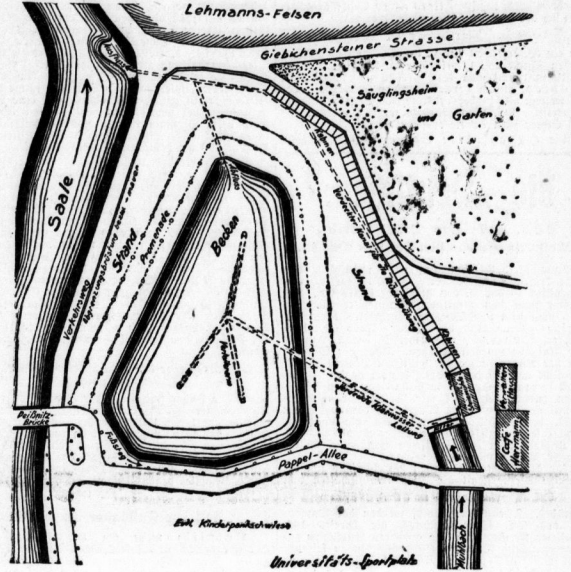
Geländeskizze zur Umgestaltung der Pregelwerke (Zeichnung 2)
