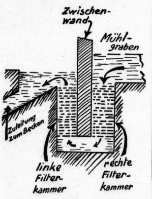
Der Schnellfilter im Durchschnitt (Schematische Zeichnung 1)
