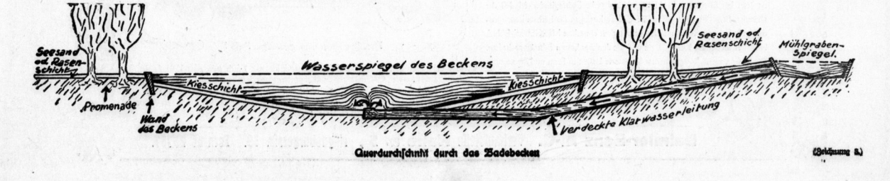
Querschnitt durch das Badbecken (Zeichnung 3)
