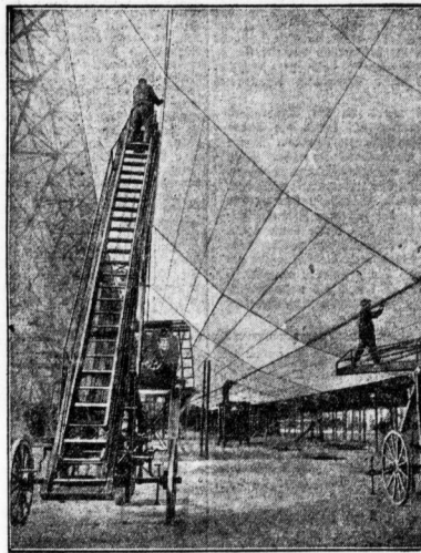
Der 285 m lange und 39,5 m hohe Luftschiffkörper, der 105 000 cbm Auftriebsgas fassen kann.
