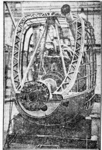
Eine der Motorgondeln mit dem Maßstab-Propellor-Motor vor dem Einbau.
