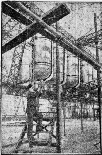
Eine Gruppe Brennstoffbehälter während der Montage im Inneren des Schiffes.
