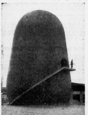
Der Trudelturbinenkanal, in dem durch senkrecht nach oben aufsteigende Luftströme Untersuchungen über den Absatz von Flugzeugen (Trudeln) durchgeführt werden
