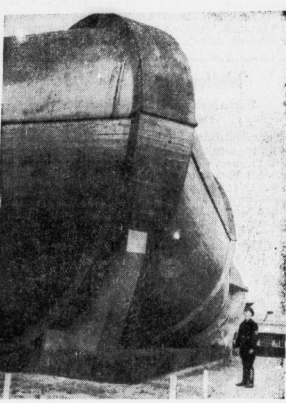
Die Außenansicht des großen Windkanals, in dem Luftströme bis zu 250 km in der Stunde erzielt werden können. Die Größe des Querschnitts erlaubt die Untersuchung von naturgetreuen Triebwerken, Leitwerken und Tragwerkteilen, sowie von Modellen bis 5 m Spannweite
