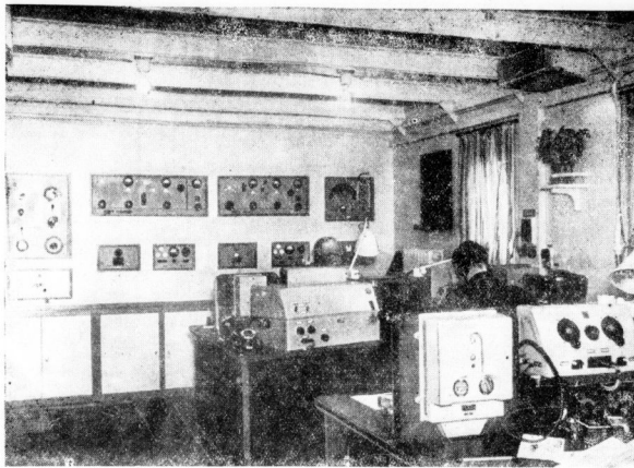
Funkraum an Bord des „Wilhelm Gustloff“. Im Hintergrund die Senderwand, rechts die Arbeitstische der Funkkollektoren mit den Empfängern.
