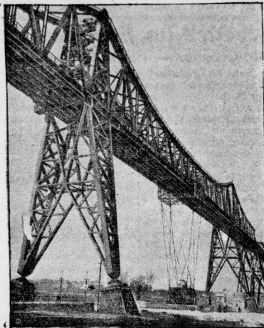
Eine der interessantesten Brückenbauten ist die Wagnbrücke über den Nordbofsee-Kanal bei Rendsburg, die zugleich mit einer Schwebefähre ausgerüstet ist.
