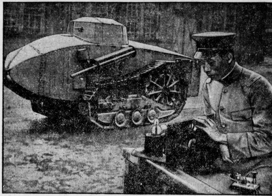
Japanischer Maschinengewehr, der aus der Ferne drahtlos gesteuert werden kann.
