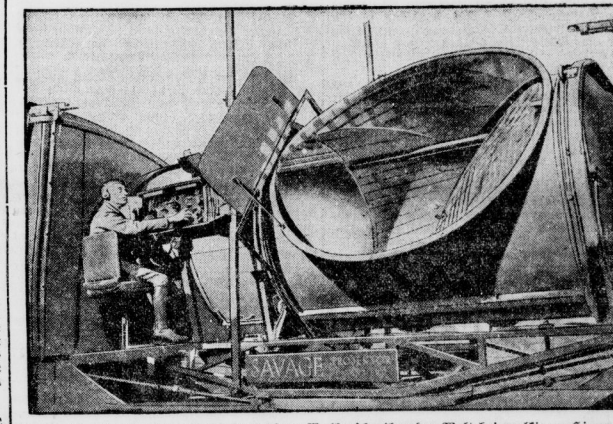
In Berlin ist der erste technisch brauchbare Wolkenschreiber der Welt bei wolkeigem Himmel in Betrieb gekommen.
