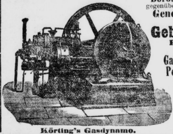
Körting's Gasdynamo.
